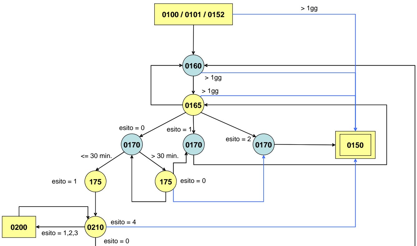
Figura 26 Sequenze dei messaggi per la gestione della richiesta del primo appuntamento per i servizi per i quali l'appuntamento è in carico all'utente del servizio di distribuzione
