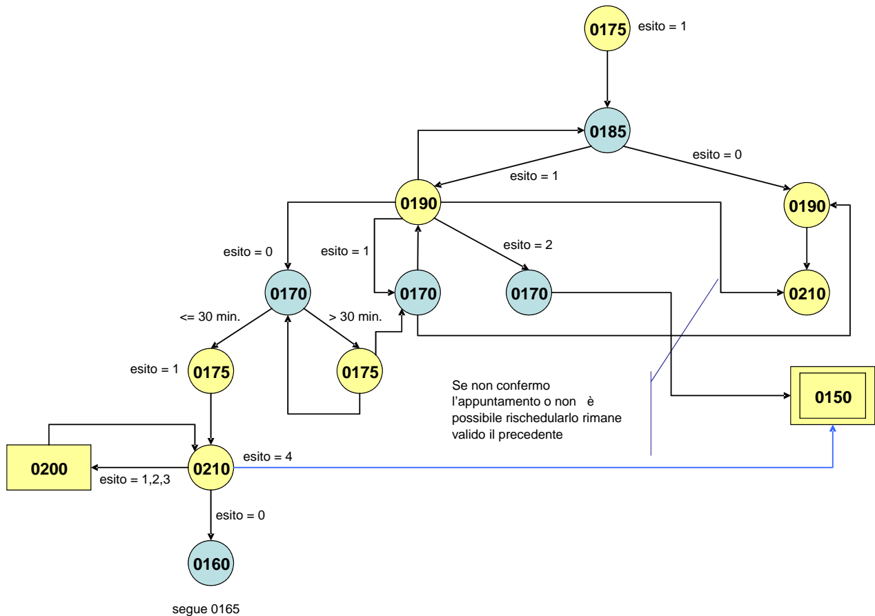
Figura 28: Sequenze dei messaggi per la gestione della modifica di un appuntamento
