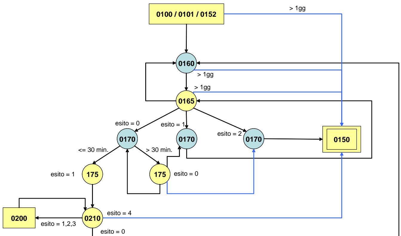
Figura 27 Sequenze dei messaggi per la gestione della richiesta del primo appuntamento per i servizi per i quali l'appuntamento è in carico all'utente del servizio di distribuzione
