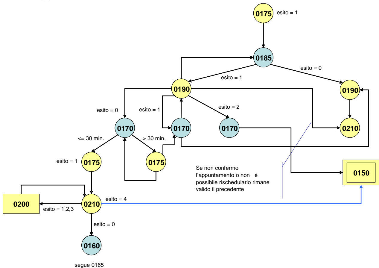
Figura 29: Sequenze dei messaggi per la gestione della modifica di un appuntamento
